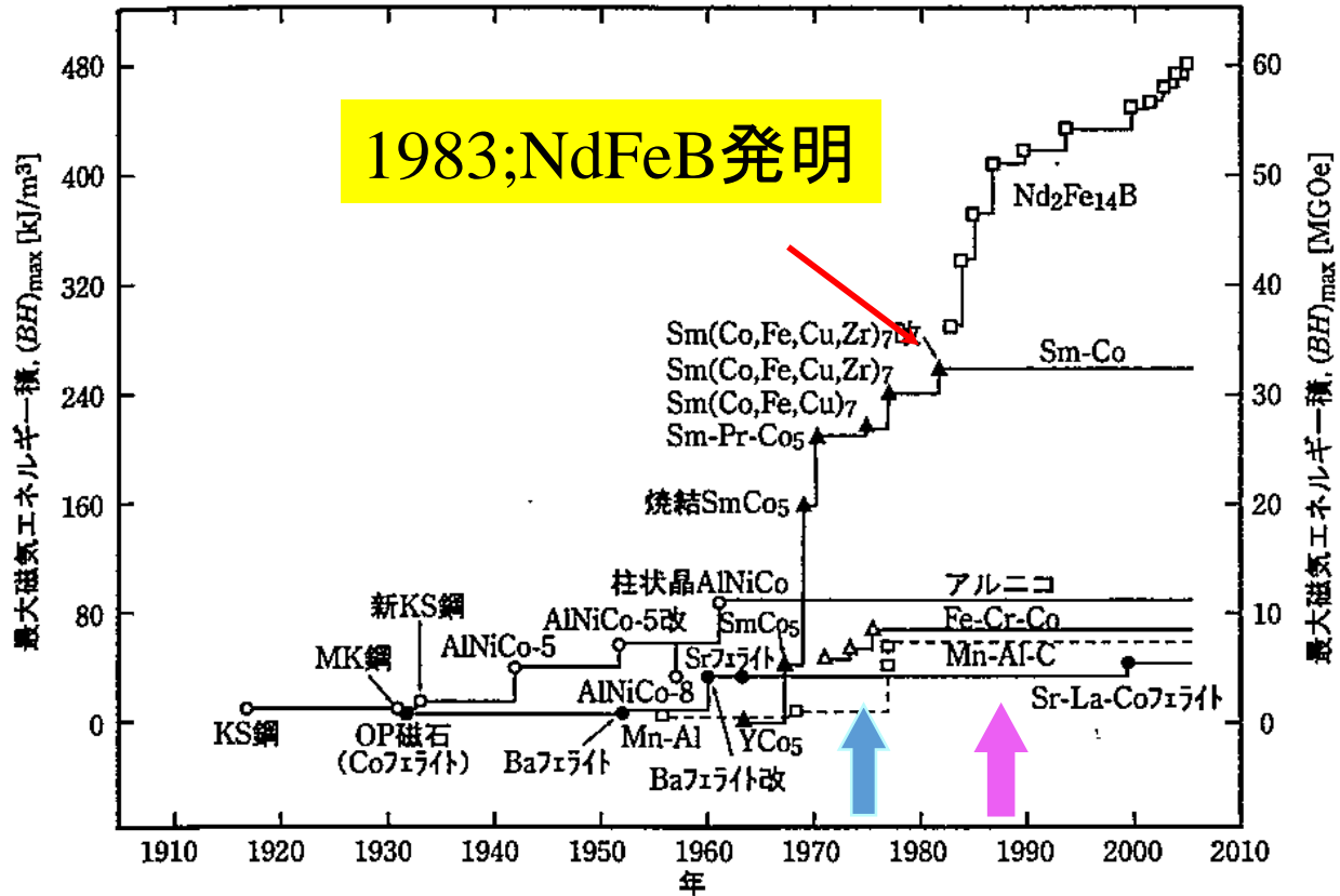
図 2.2 永久磁石の最大磁気エネルギー積 (BH)_{max} の推移
